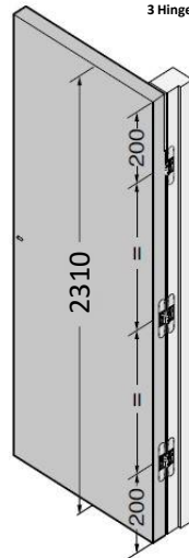
B 3 symmetrisch angeordnete Bänder / 3 Scharnieren symmetrisch verdeckt / 3 Hinges arranged symmetrically
