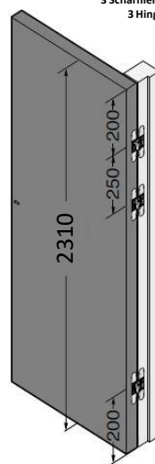
C 3 asymmetrisch angeordnete Bänder / 3 Scharnieren asymmetrisch verdeckt / 3 Hinges arranged asymmetrically
