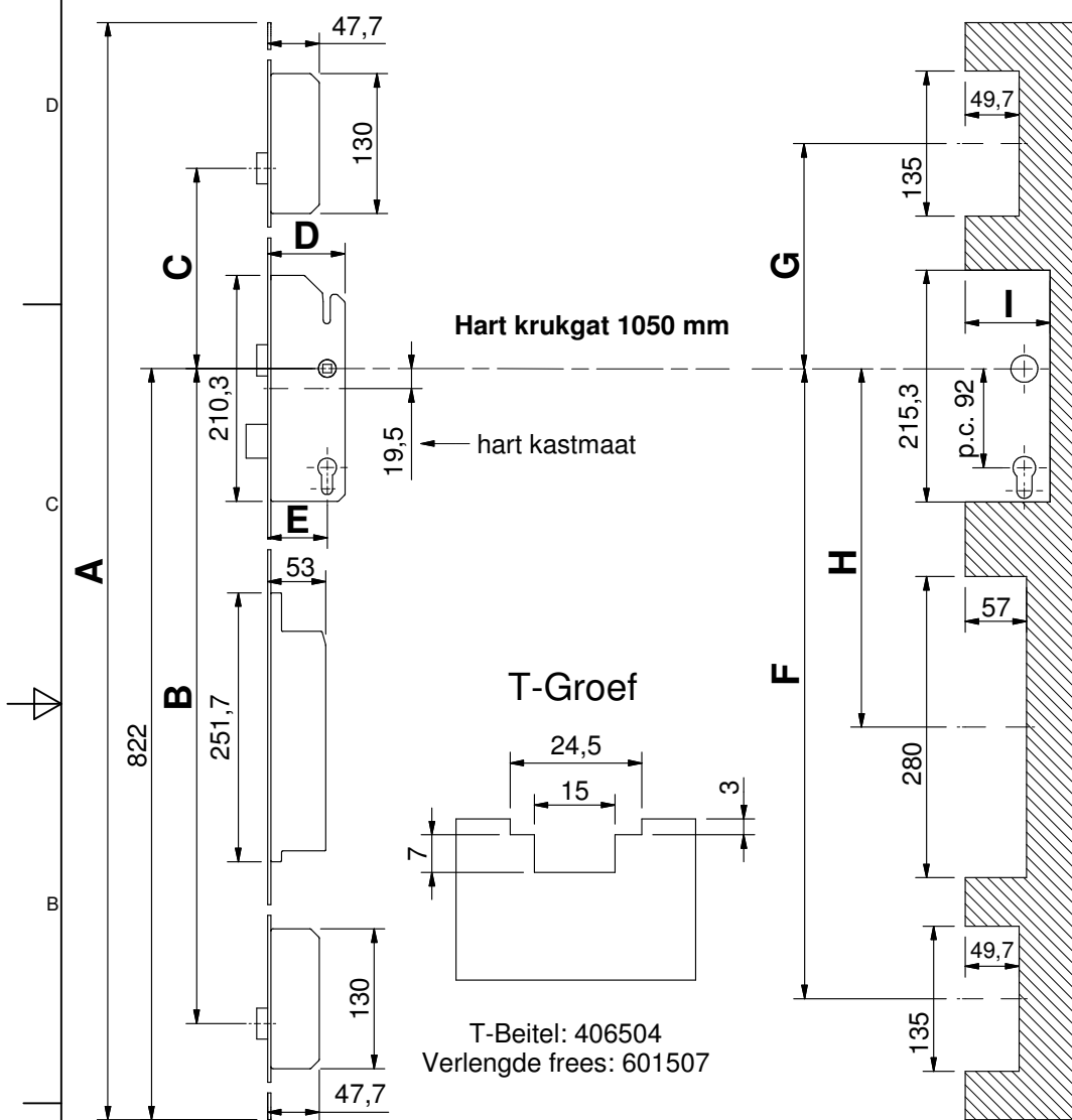
Overzicht afmetingen Automotortronic
