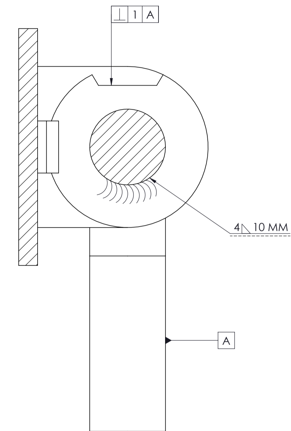
DOORSNEDE A-A SCHAAL 2:1
