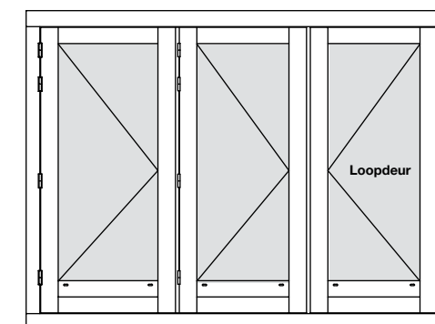
Afb. 3 Optie 3 (scharnierzijde)
