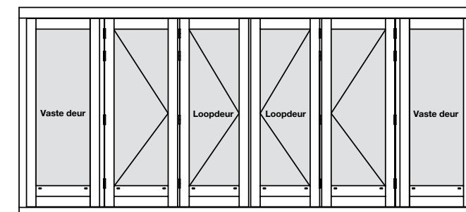
Afb. 1 Optie 1 (scharnierzijde)
