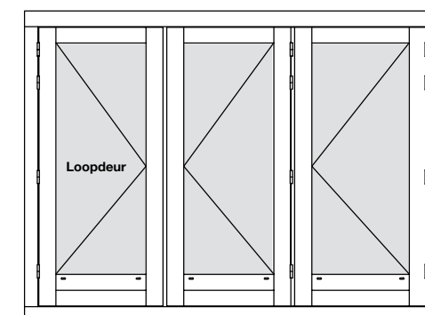
Afb. 4 Optie 4 (scharnierzijde)
