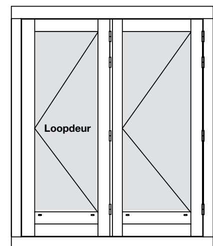
Afb. 8 Optie 8 (scharnierzijde)
