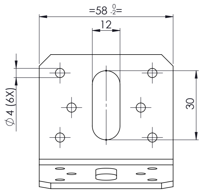
AANZICHT A
