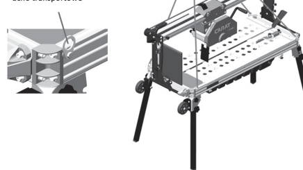
ucho transportowe
