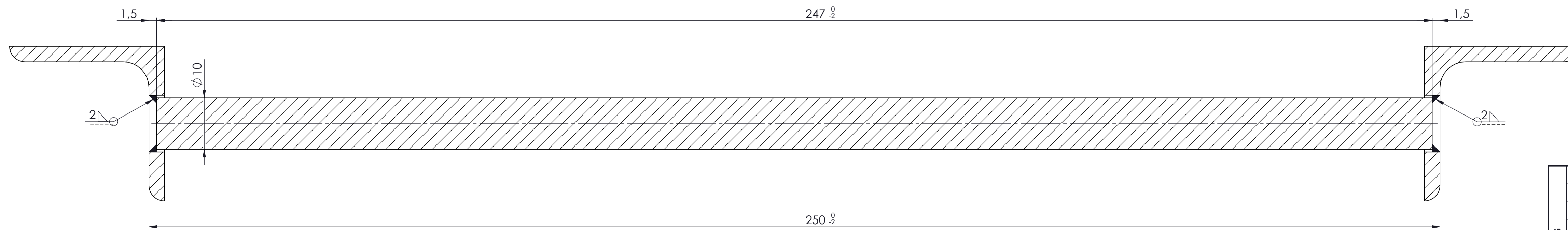
DOORSNEDE A-A SCHAAL 2:1
