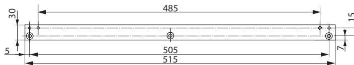
Vlakte montageplaat A115 voor glijarm G461.
