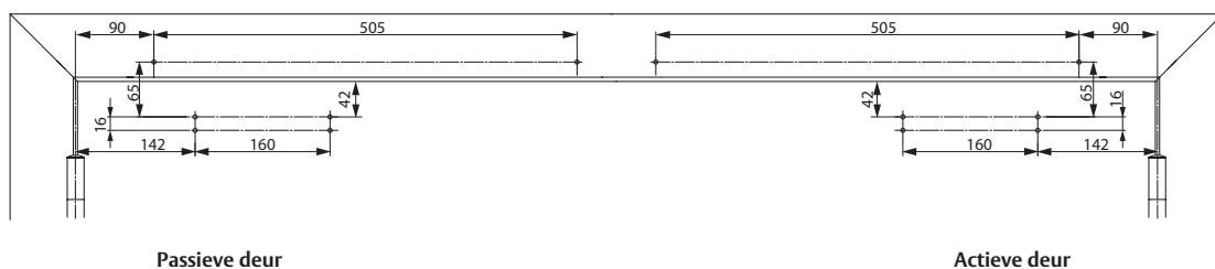
Montage configuratie deurblad scharnierzijde
