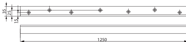
Hoekmontageplaat A117 middensteun voor montage van glijarm G461 op niet-scharnierzijde.
