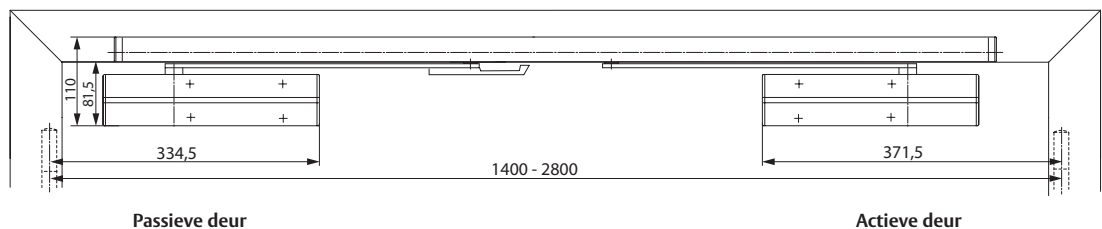
2 - Deurbladmontage niet-scharnierzijde
