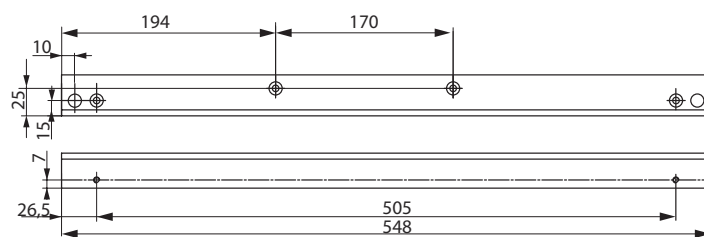
Hoekmontageplaat A116 voor montage van glijarm G461 op niet-scharnierzijde.
