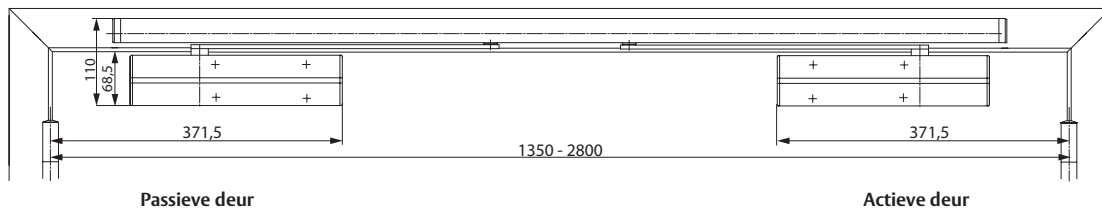
1-Deurbladmontage scharnierzijde
