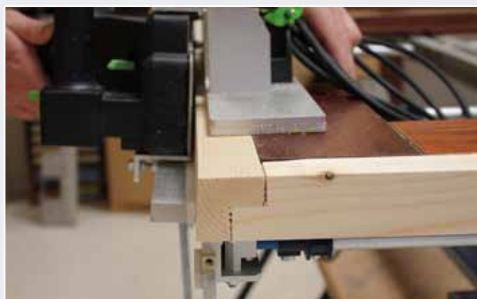
Afb. 25 Afschaven zijkant
