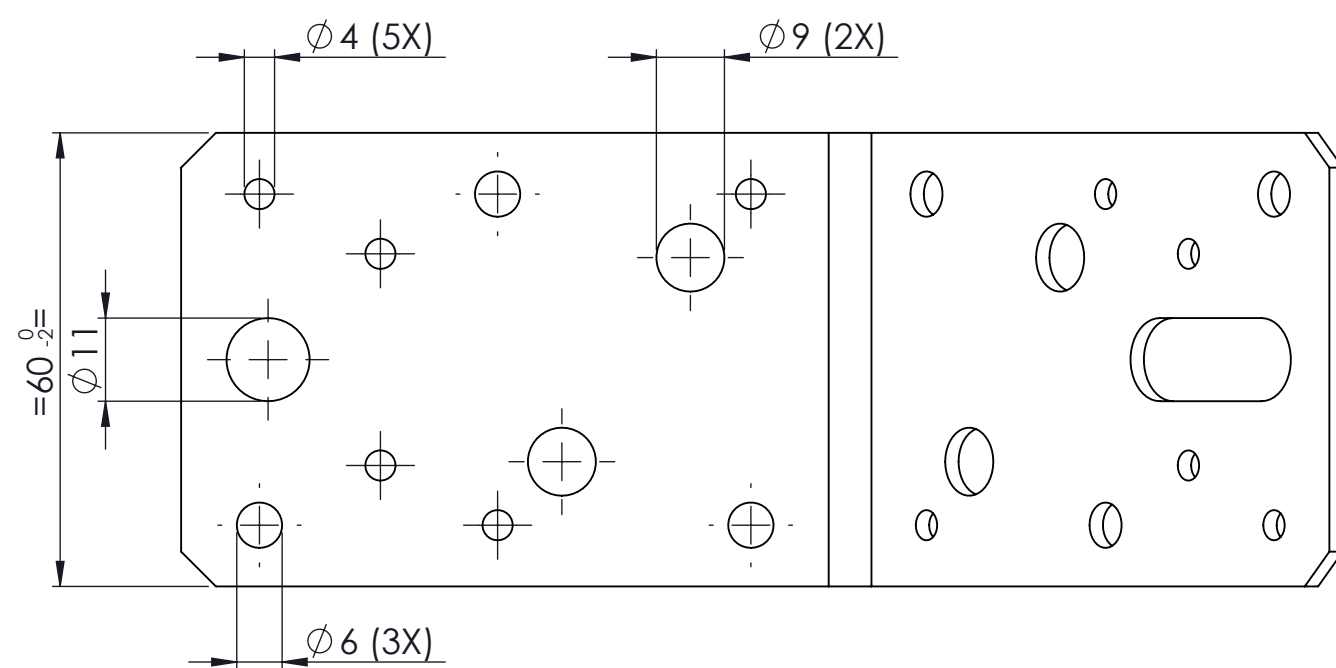
AANZICHT A
