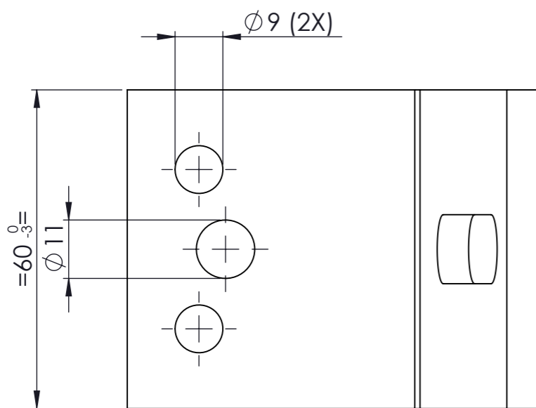
AANZICHT A 90° GEDRAAID
